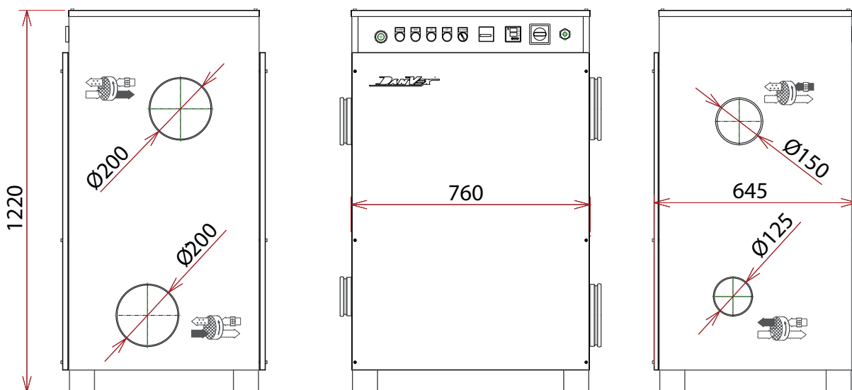
Рис 2. Размеры осушителя воздуха AD-800
