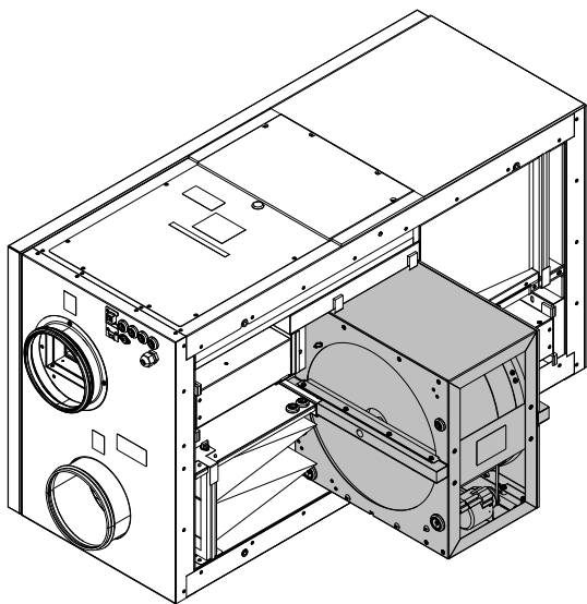
Рис. 4 теплообменник
