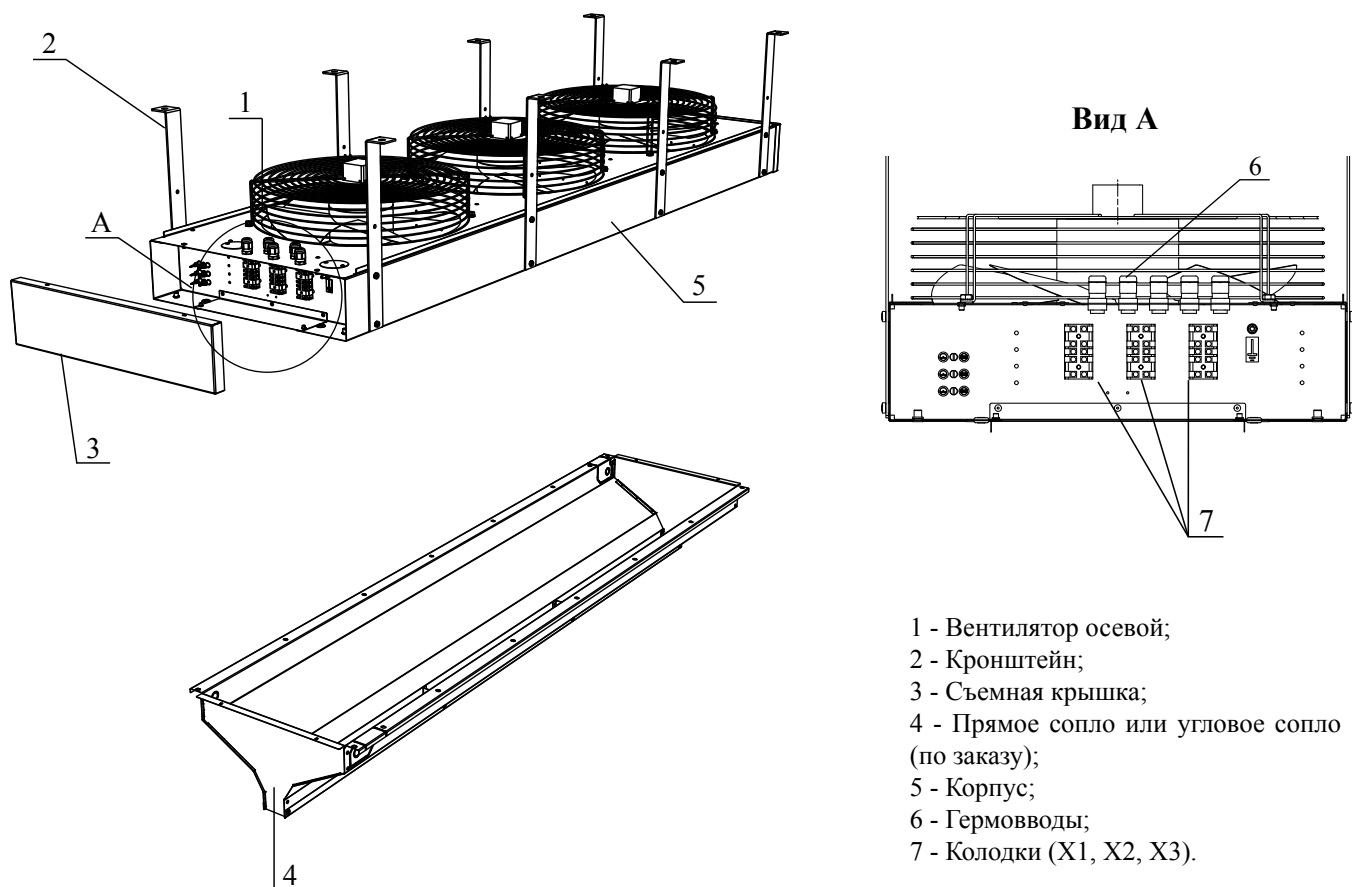
Рисунок 1. Воздушная завеса
