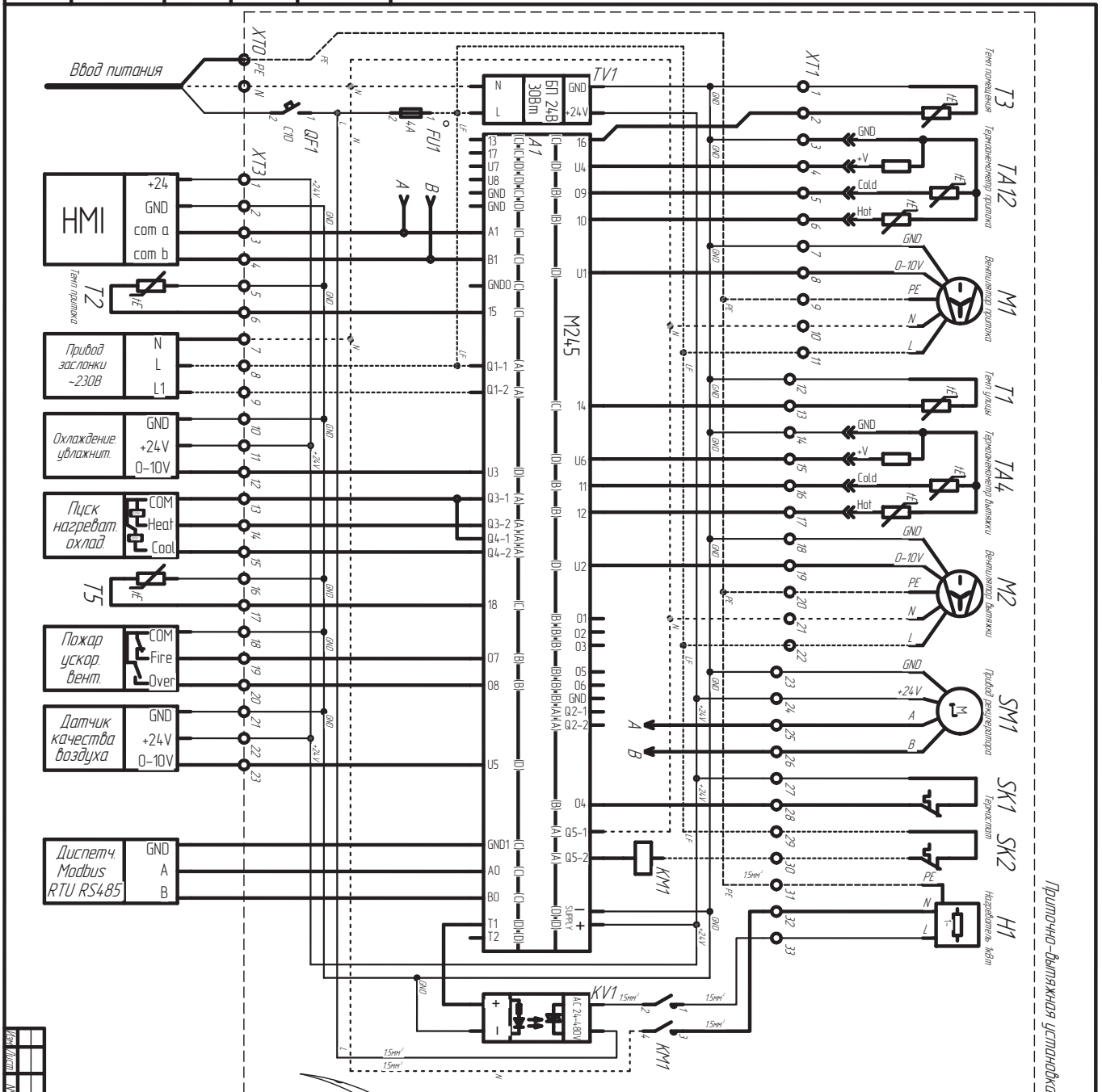
Блок клемм XT13 (для внешних подключений)
