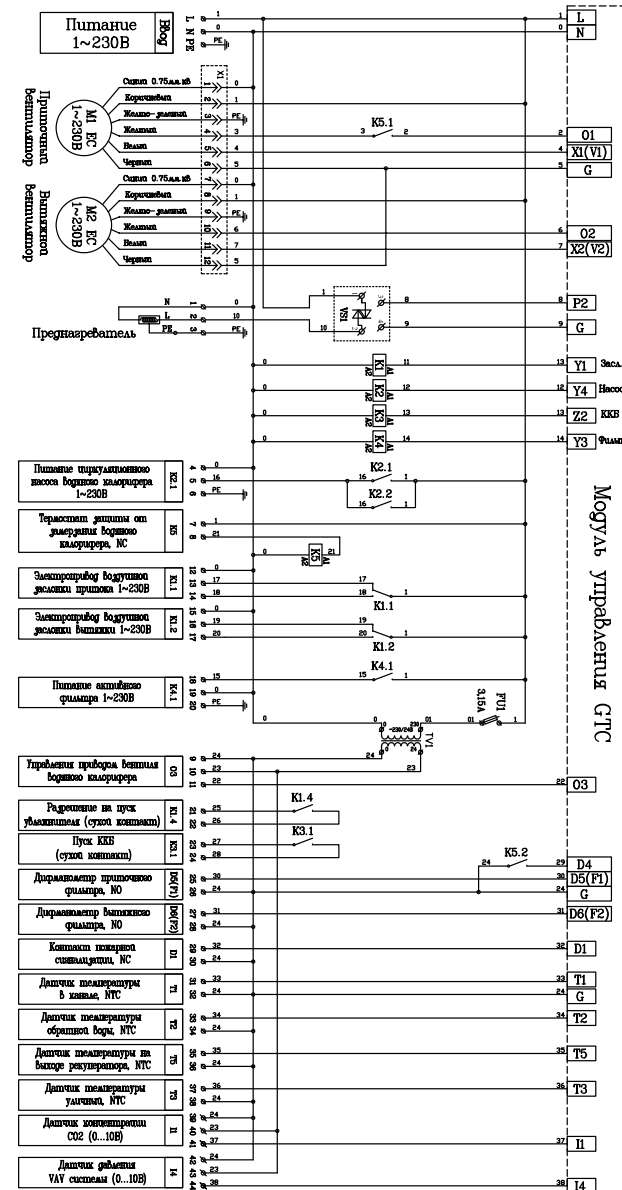
Схемы подключения ZPVP 450 PW EC, ZPVP 850 PW EC
