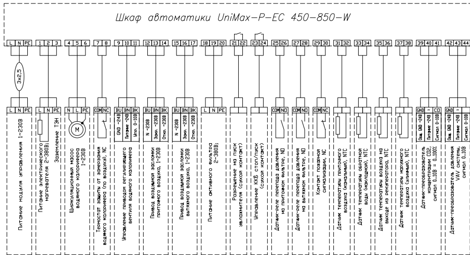
Схемы подключения ZPVP 450 PW EC, ZPVP 850 PW EC
