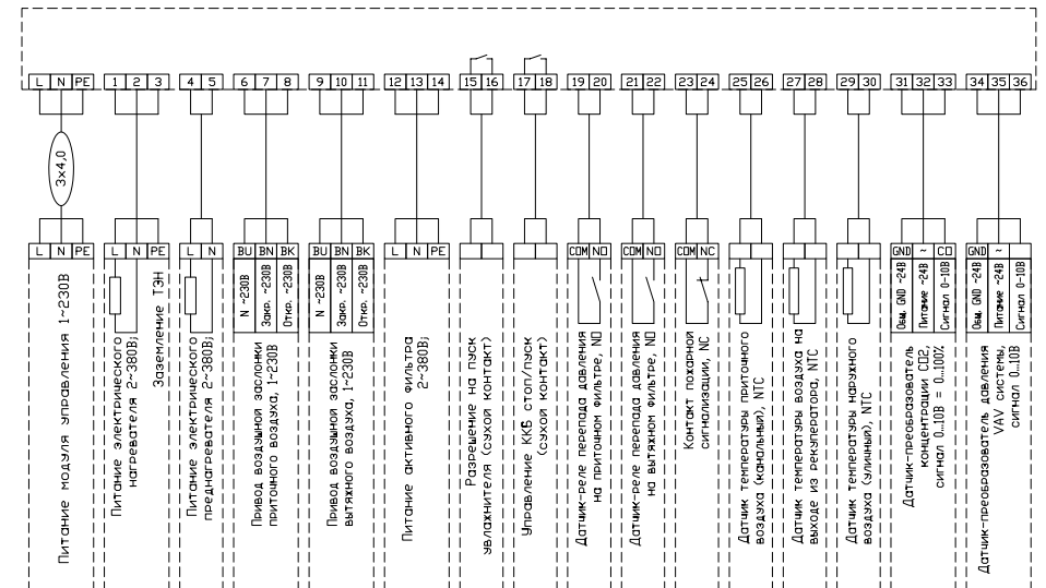
Схема подключения ZPVP 450 PE EC, ZPVP 850 PE EC
