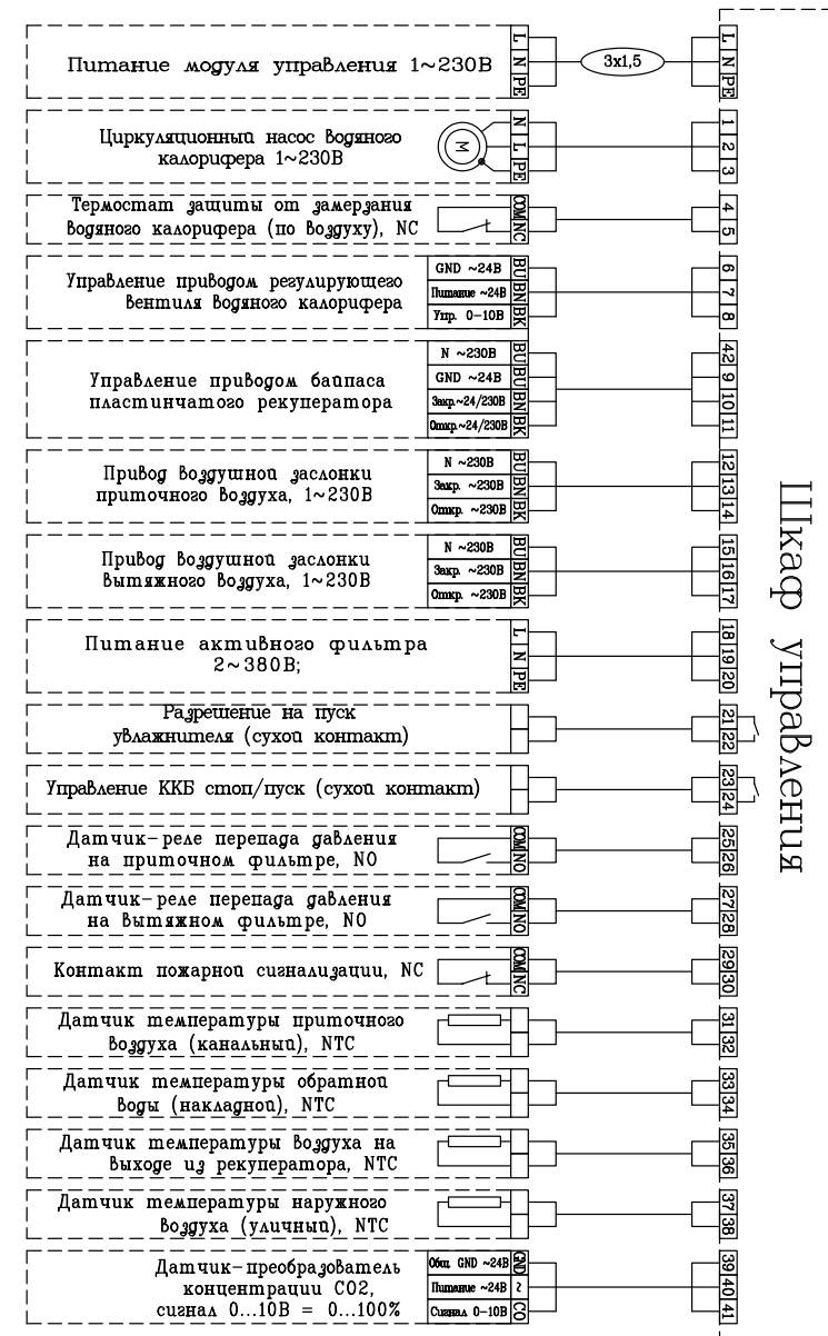
Схема ZPVP 1000 PW, ZPVP 1500 PW
