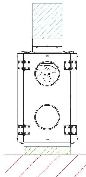
Вид слева
