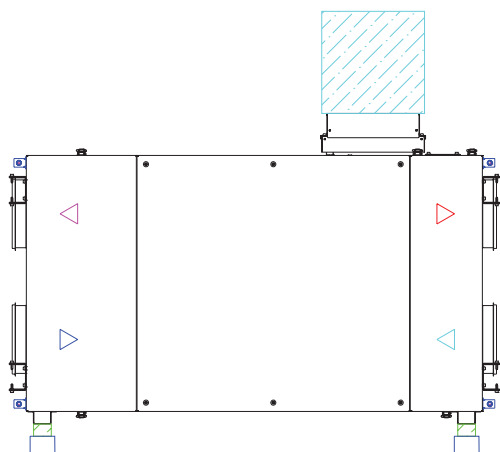
Главный вид
