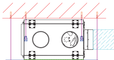
Вид слева
