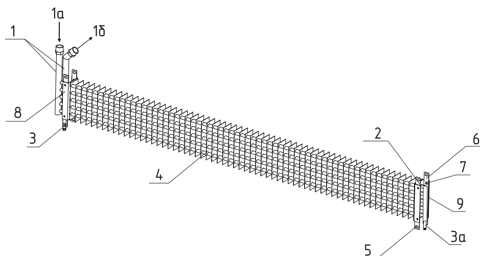
Рис. 2. Водяной воздушнонагреватель
