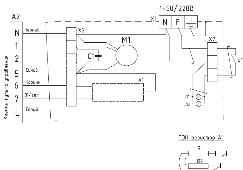
Рис. 7. КЭВ-110П6130W, КЭВ-110П6150W
