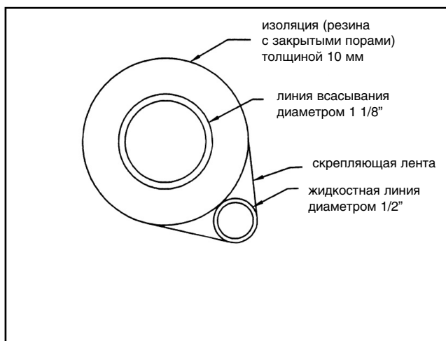
Рис. 9 Теплоизоляция труб
