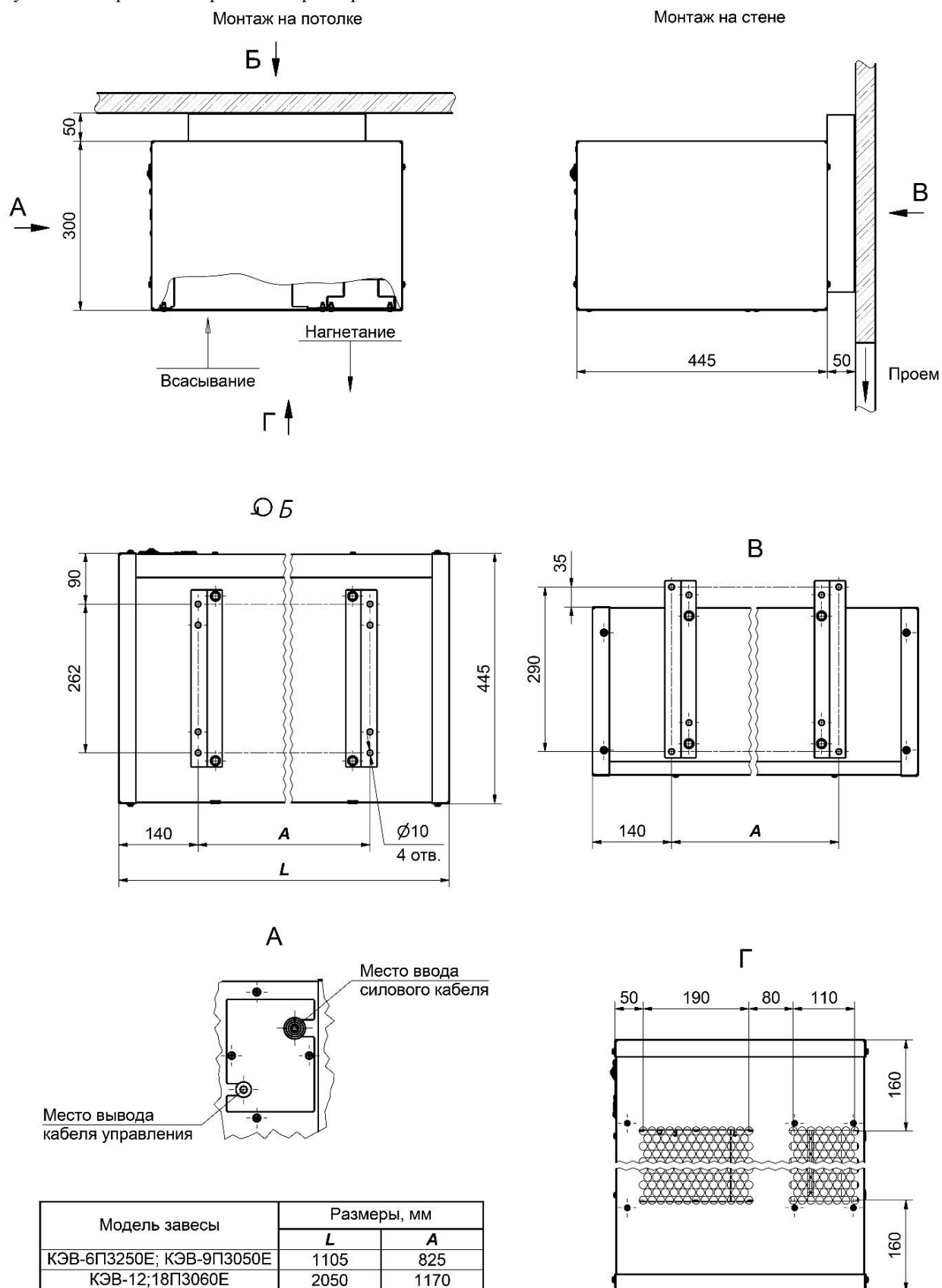
Рисунок 1-Габаритные и крепежные размеры
