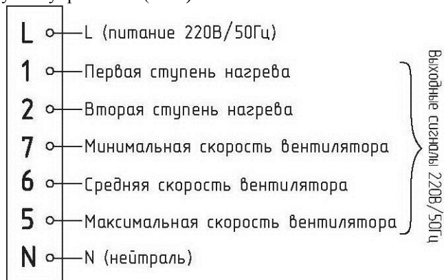
Рисунок 5-Назначение клемм пульта управления (IR03)
