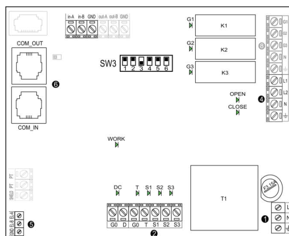
ПЕЧАТНАЯ ПЛАТА ВОЗДУХОНАГРЕВАТЕЛЯ
