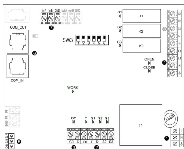
ПЕЧАТНАЯ ПЛАТА ЗАВЕСЫ
