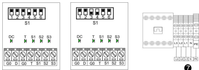
ПЕЧАТНАЯ ПЛАТА ВОЗДУХОНАГРЕВАТЕЛЯ
