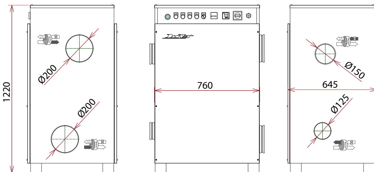
Рис 2. Размеры осушителя воздуха AD-800
